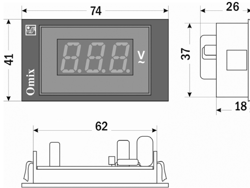
Рис. 3 – Размеры прибора
