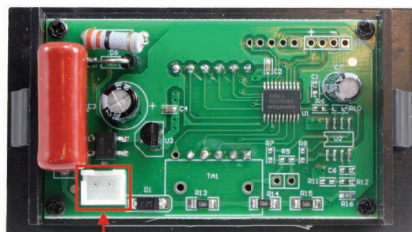
Разъем 2pin для входного сигнала и питания
